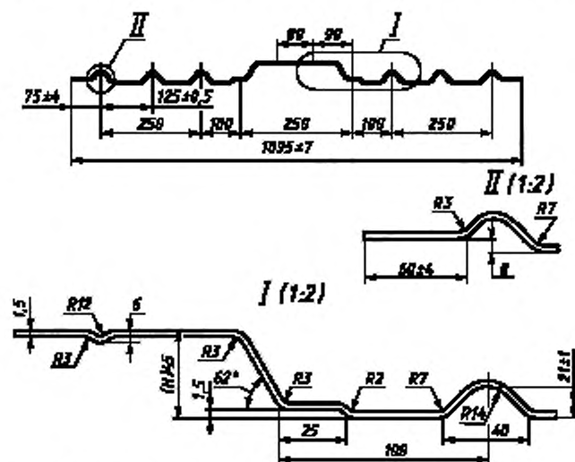
Рисунок 2 — Профиль 1095-45-21-1,5, ГЛ4-220А
