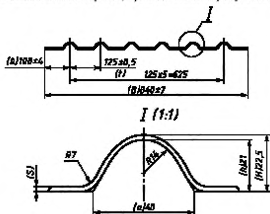
Рисунок 1 — Профиль 840-21-1,5, ГЛ4-218; профиль 840-21-2,0, ГЛ4-219
